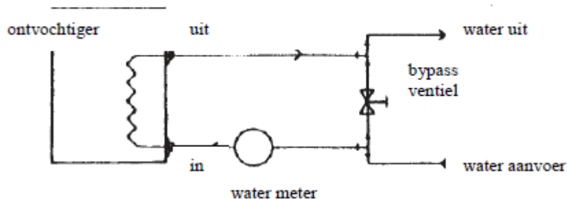
Рис.8. осушитель Драйфаст (DHW) с рекуперацией тепла в воду.
