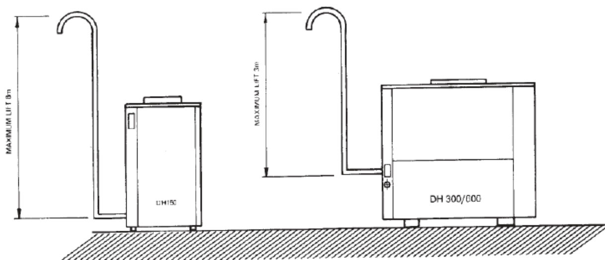
Рис.9. осушитель Драйфаст с водяной помпой для принудительного отвода конденсата. Устанавливается в случае, когда осушитель находится ниже канализационного слива, (наружная установка для DHW 300 и внутренняя для моделей DHW150, DHW600).
